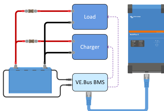
Het VE.Bus BMS NG schakelt belastingen en laders uit via de "belastingontkoppeling" en "laadontkoppeling" en regelt de omvormer/acculader.
