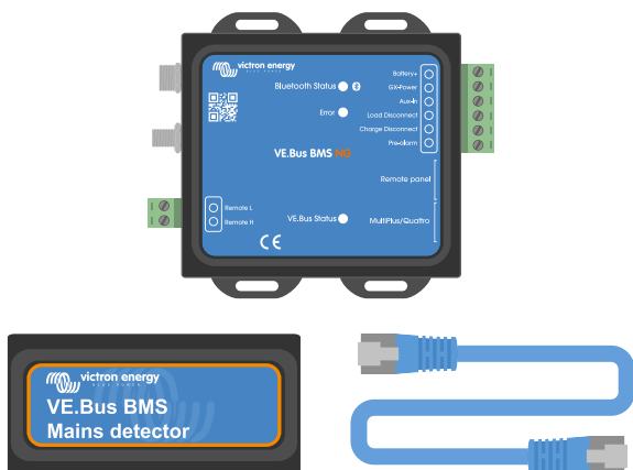
VE.Bus BMS NG, VE.Bus BMS-netdetector en RJ45 UTP-kabel.
