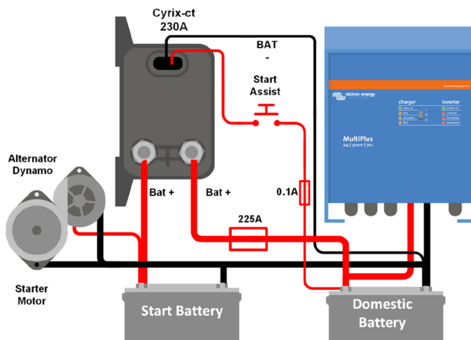
Cyrix-ct 12/24-230: aansluitschema
